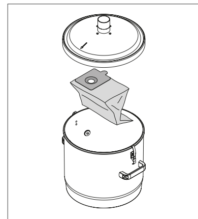
Esploso del sistema di filtrazione
